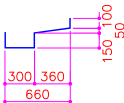
DETALHE DA CALHA
